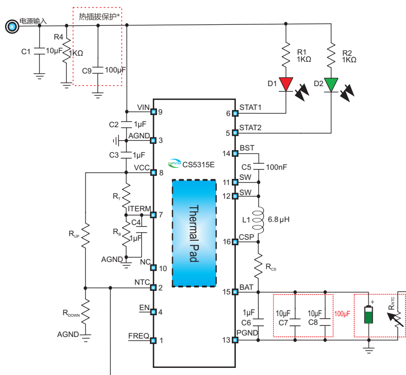
CS5315E应用电路图
