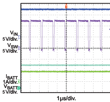
En On V_{BATT} = 10.8V
