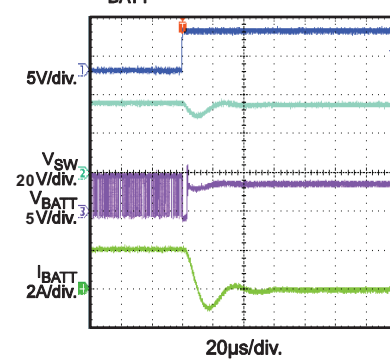
En Off V_{BATT} = 10.8V
