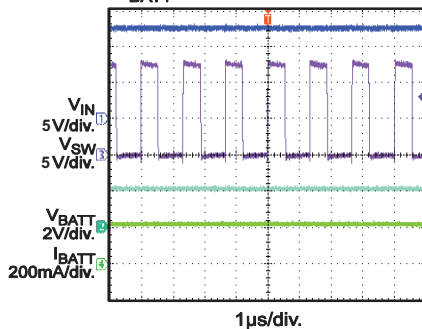
CV Steady State V_{BATT} = 12.6V
