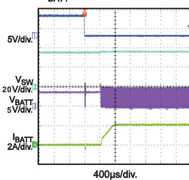
En On V_{BATT} = 10.8V
